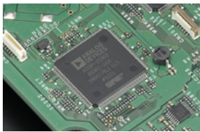
Per la IF principale DSP, unità di trasmissione ADSP-21363 clock @333 MHz
