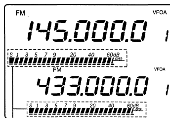
S-meter durante la ricezione Indicatore di potenza RF durante la trasmissione
