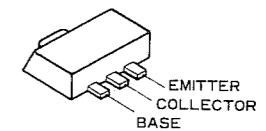
2SB799(ML) (Q4001, 4007)
