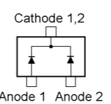
DAN222 (N) (D4006, 4008)
