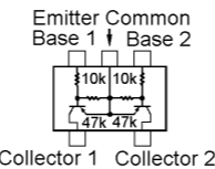
UMA8N (A8) (Q4008, 4010)
