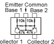
UMA8N (A8) (Q4008, 4010)
