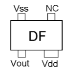
PST3445UR (DF) (Q4014)
