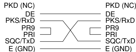
Connettore DATI
