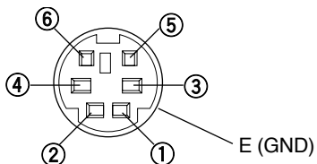
Connettore DATI
